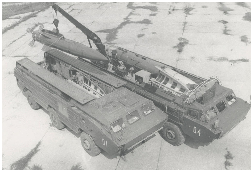
Заряжание тактического ракетного комплекса «Точка»
